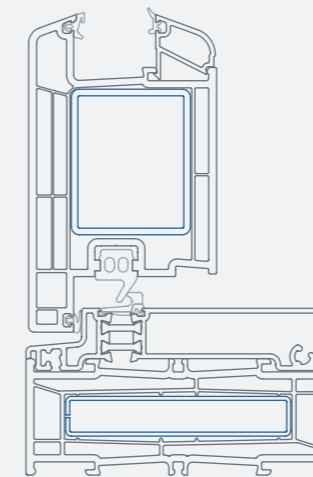
Deur NL71 Arcade naar buiten draaiend
