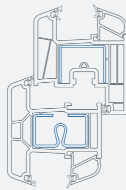
T- Kozijnprofiel
