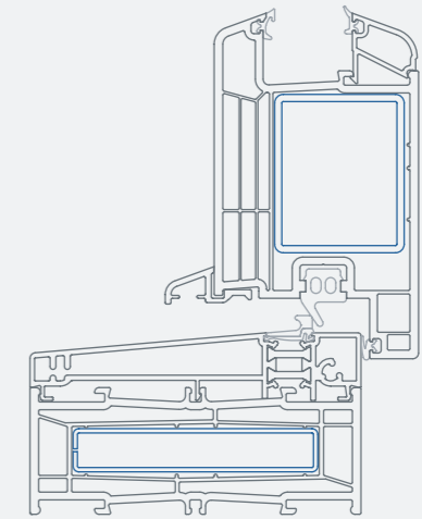
Deur NL71 Arcade naar binnen draaiend
